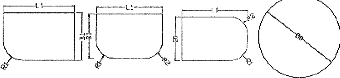
Zuschnitt 25 mm Links vorne angerundet
