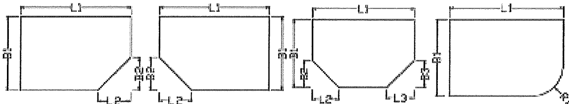
Zuschnitt 25 mm Rechts vorne abgeschrägt
