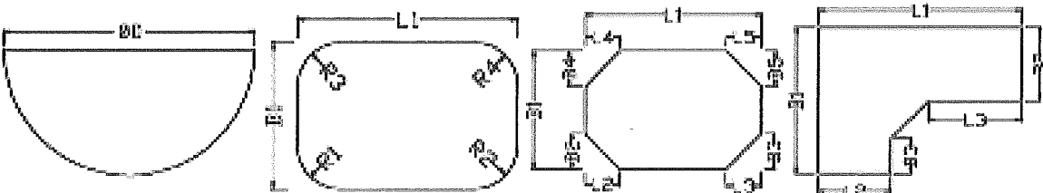
Zuschnitt 25 mm halb Kreis
